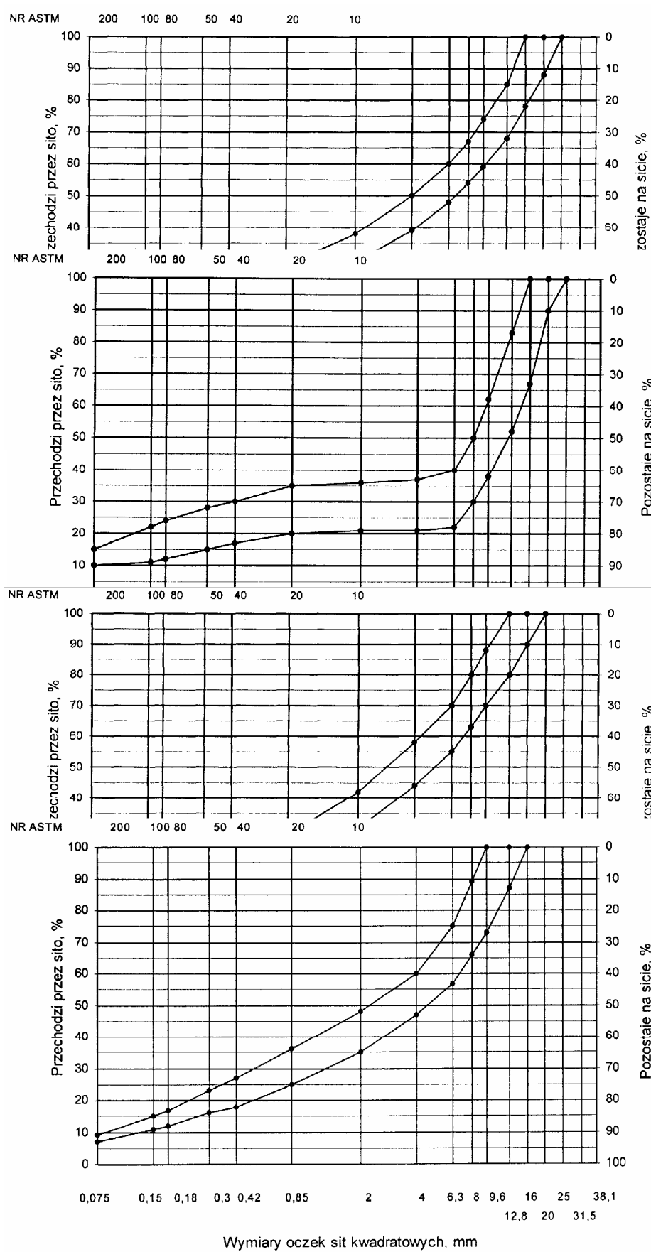
Rys. 4. Krzywe graniczne uziarnienia mieszanki mineralnej BA od 0 do 20 mm do warstwy ścieralnej nawierzchni drogi o obciążeniu ruchem od KR3 do KR6
