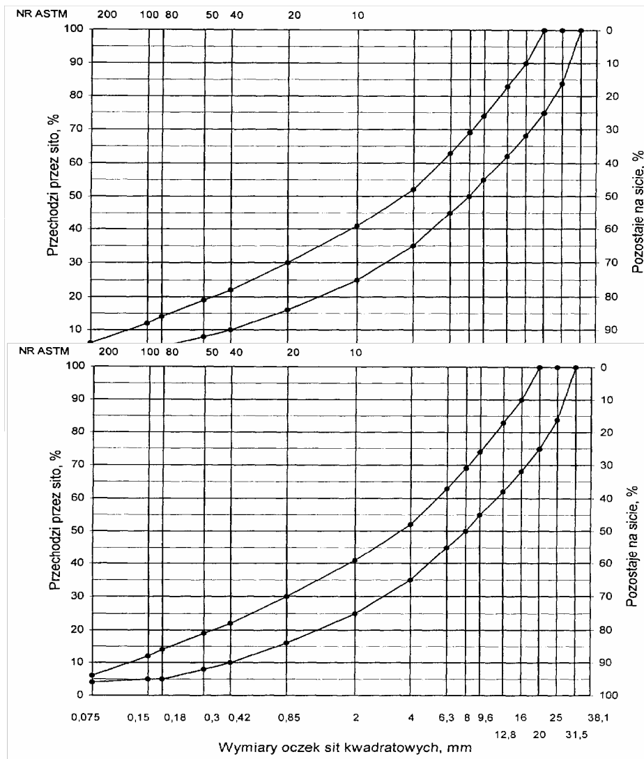
Rys. 11. Krzywe graniczne uziarnienia mieszanki mineralnej BA od 0 do 25 mm do warstwy wiążącej, wyrównawczej i wzmacniającej nawierzchni i drogi o obciążeniu ruchem od KR3 do KR6
